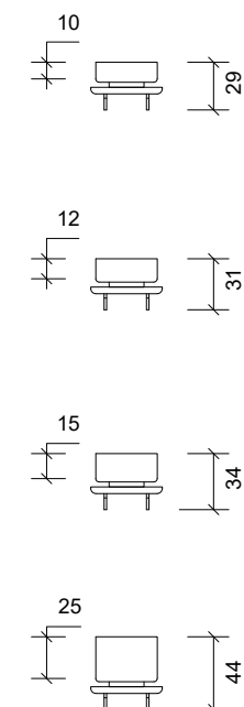
Side Opstalt/Side Elevation/Seitenansicht
