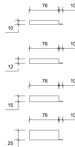
Side Opstalt/Side Elevation/Seitenansicht
