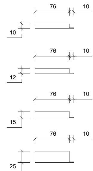
Side Opstalt/Side Elevation/Seitenansicht
