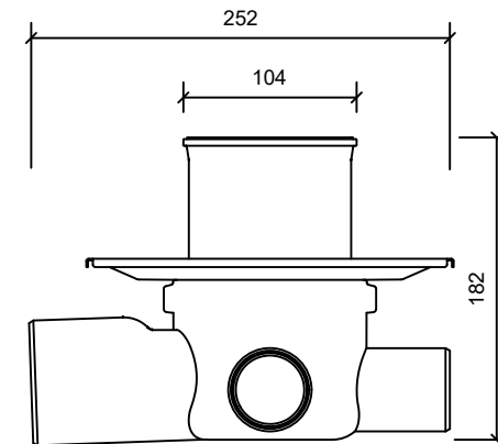
Side Opstalt/Side Elevation/Seitenansicht
