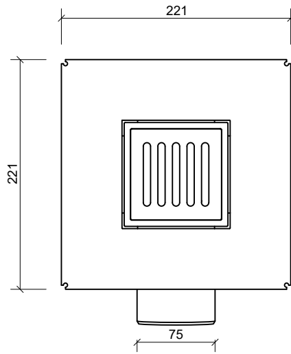
Plan/Plan/Draufsicht
