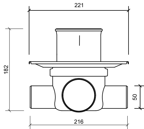
Front Opstalt/Front Elevation/Frontansicht
