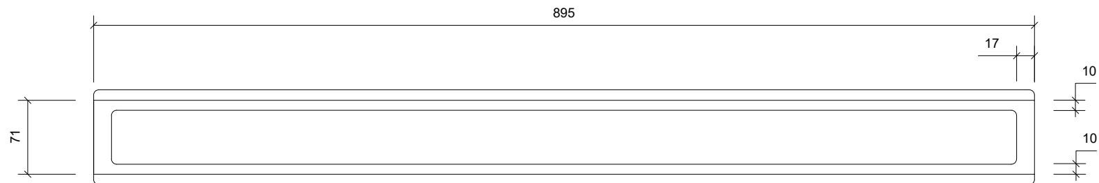
Plan/Plan/Draufsicht
