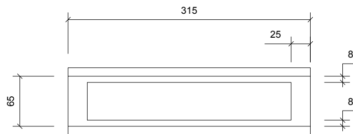
Plan/Plan/Draufsicht
