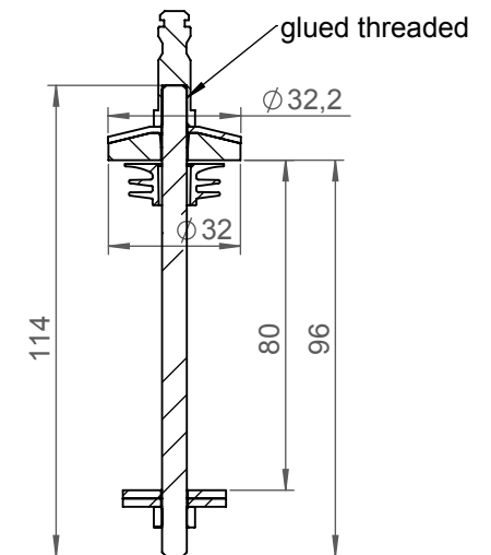
SCHNITT A-A
