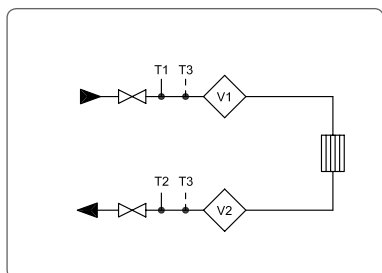
Eksempel 1: Lukket termisk system med en eller to flowmålere
