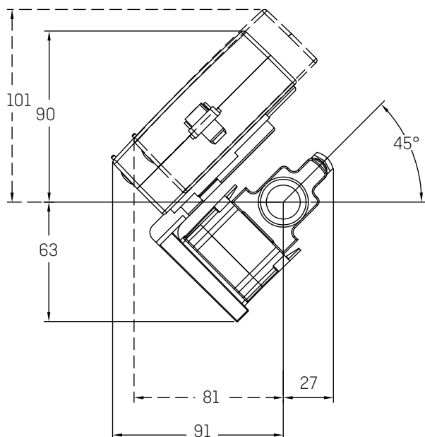
MULTICAL® 602 frontmål
