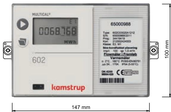
Panelmonteret MULTICAL® 602 set forfra
