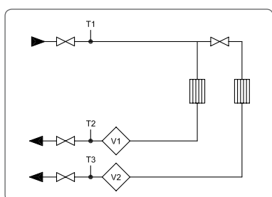
Eksempel 3: To varmekredse med fælles fremløb
