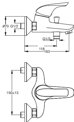
Kar-/brusebatteri Varenr.: B 3697 AA
