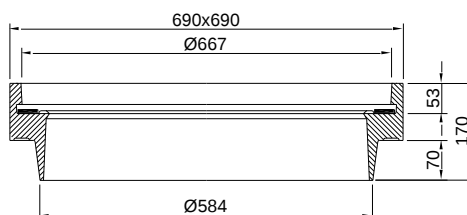
Ø600 Firkantkarm
