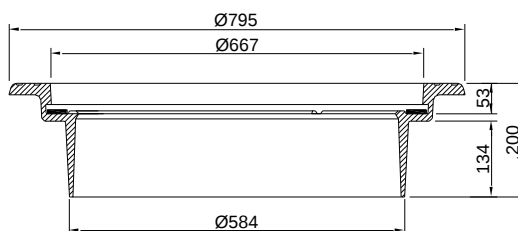
Ø600 Flydekarm Med inspektionsslidser. 320 mm. ved langt skørt
