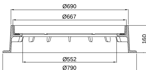
Ø600 Fast karm 16 cm
