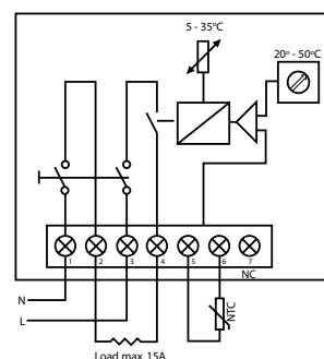
Koblingsdiagram DEVlreg™ 532
