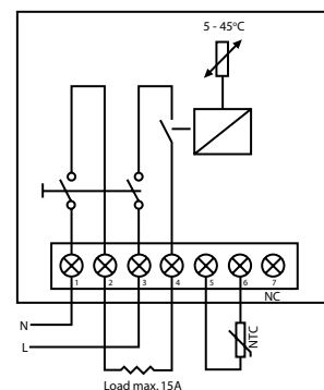
Koblingsdiagram DEVlreg™ 530
