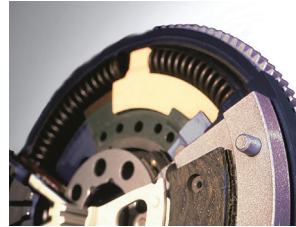
Resortes para embragues: alta resistencia a la deformación por fuerzas laterales y bajo peso
