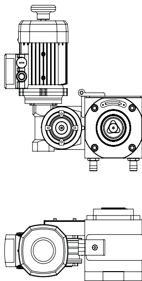
VERSIONE DI MONTAGGIO V1 - L1 ASSEMBLY VERSION V1 - L1
