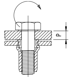
COPPIA DI SERRAGGIO MASSIMA MAX TORQUE
