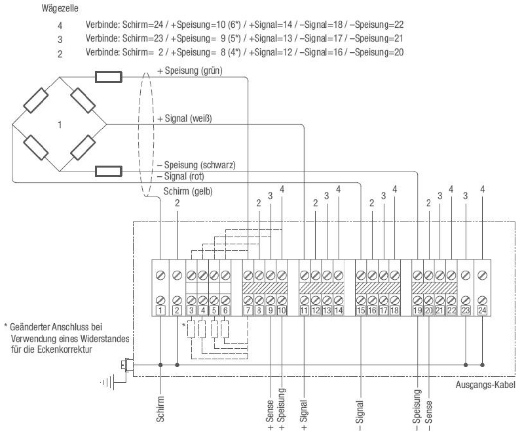
Abbildung 2: Kabelanschluss
