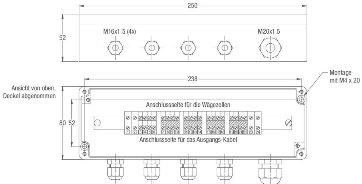
Abbildung 1: Abmessungen in [mm]
