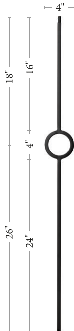
9050VS 10 pcs per box 540 pcs per skid
