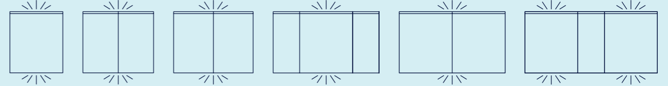
B60 • H70 • D12 B80 • H70 • D12 B90 • H70 • D12 B120 • H70 • D12 B120 • H70 • D12 B150 • H70 • D12
