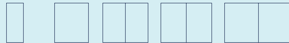
B30 • H70 • D12 B60 • H70 • D12 B80 • H70 • D12 B90 • H70 • D12 B120 • H70 • D12
