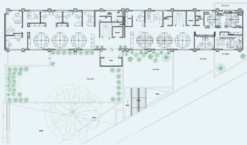
Planta Primer Nivel
