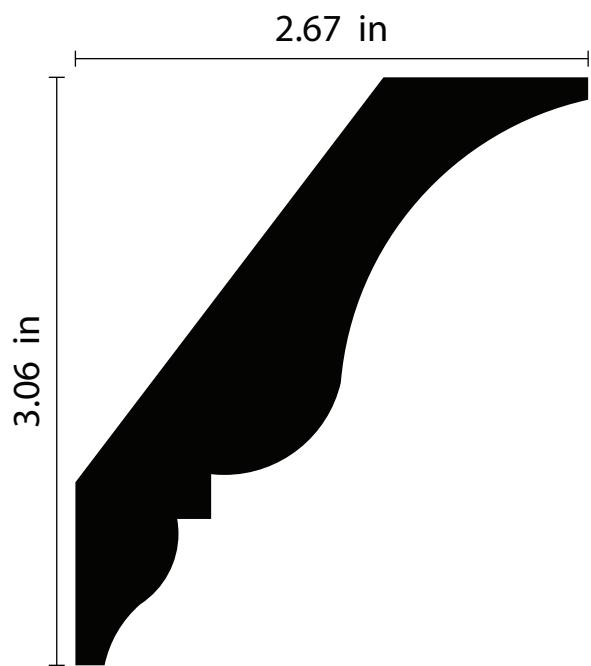
CN-103 .84" x 4.00"
