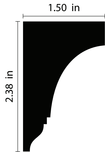
CN-121 1.5" x 2.375"
