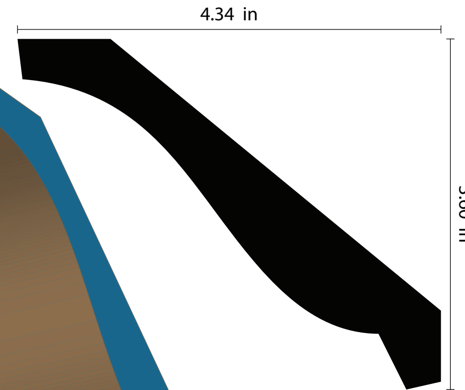
CN-056 1.0" x 5.687"
