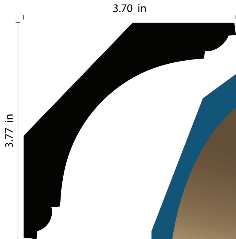
CN-080 1.4375" x 4.20"
