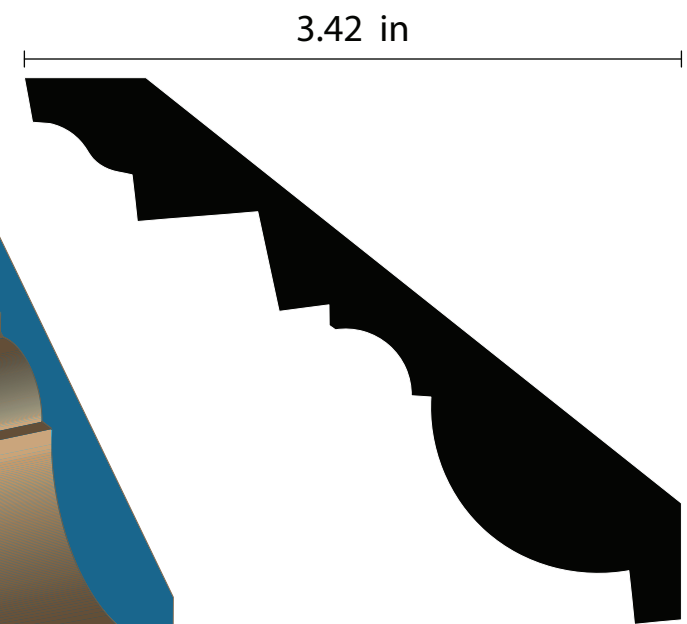
CN-007 .75" x 4.5"
