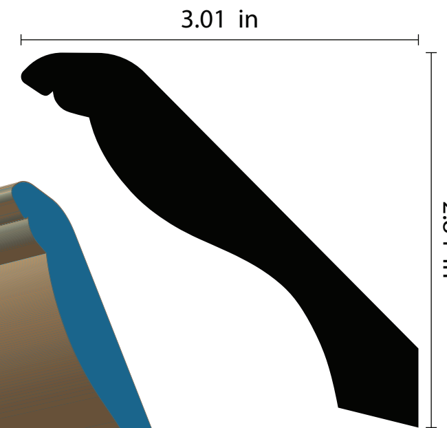
CN-095 0.75" x 4.00"
