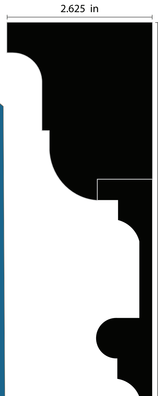
CN-113 2.63" x 6.75"
