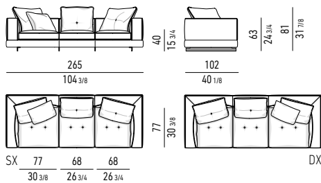
LOW DIVANO ANGOLARE CM 265 LOW CORNER SOFA CM 265
