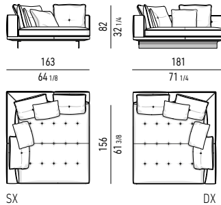
CHAISE-LONGUE CM 163X181 CHAISE-LONGUE CM 163X181
