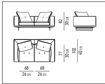
MODULO DI SEDUTA CM 68 SEAT CUSHION CM 68
