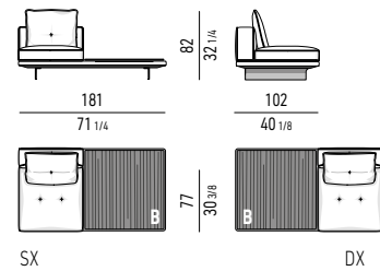
ELEMENTO CENTRALE CM 181 CON TOP B CENTRAL ELEMENT CM 181 WITH TOP B
