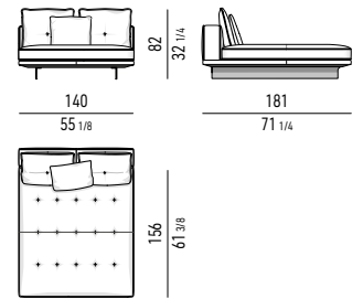
DOPPIO COUCH CM 140X181 DOUBLE COUCH CM 140X181
