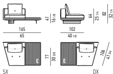
ELEMENTO CENTRALE ASIMMETRICO THEATRE CM 165 CON TOP E THEATRE ASYMMETRICAL CENTRAL ELEMENT CM 165 WITH TOP E
