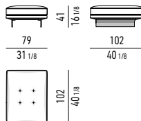
POUF CM 79X102 OTTOMAN CM 79X102
