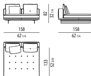
DOPPIO COUCH CM 158X158 DOUBLE COUCH CM 158X158
