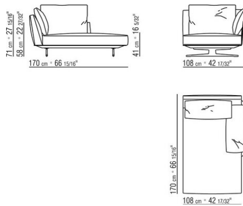
COD. 029021 LONG CORNER L
