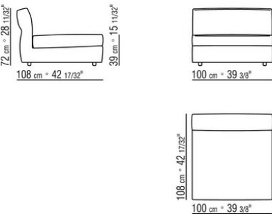
COD. 024313 UNIT / SOLOTEX
