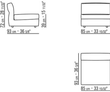
COD. 024305 UNIT
