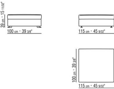
COD. 024356 OTTOMAN SOLOTEX
