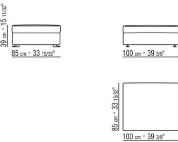
COD. 024355 OTTOMAN SOLOTEX
