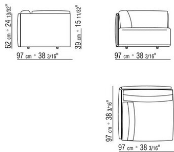
COD. 015Z35 LONG CORNER L
