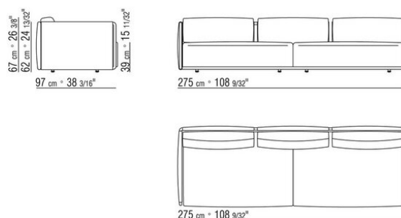
COD. 015Z23 END UNIT L
