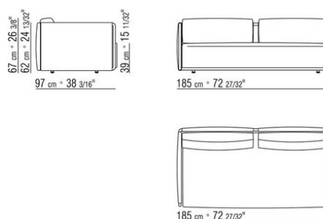
COD. 015Z25 END UNIT L
