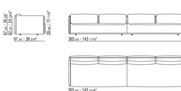
COD. 015Z25 END UNIT L
