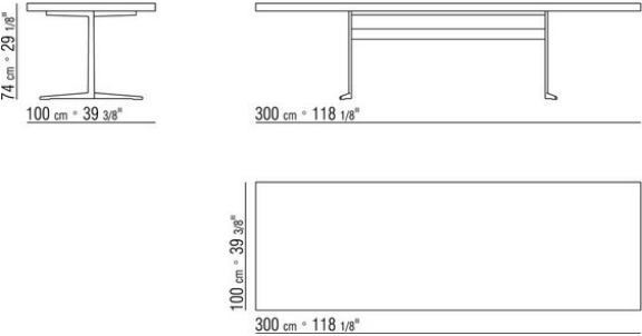
COD. 014X72 TABLE
