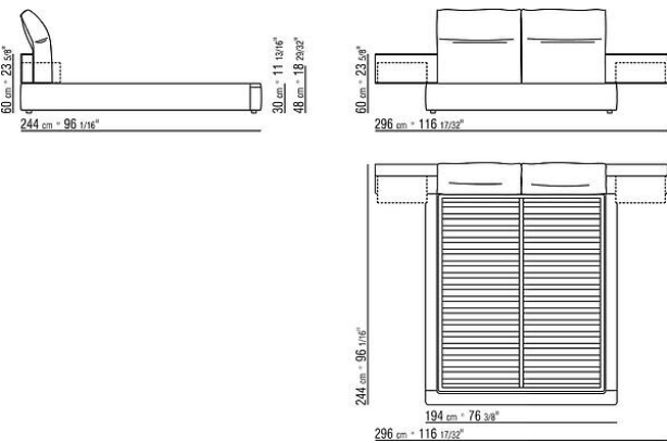
COD. 0243Q2 BED W/ SLATS
