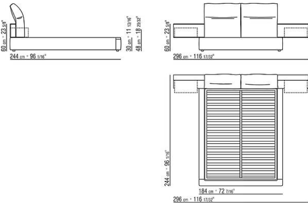
COD. 0243Q1 BED W/ SLATS
