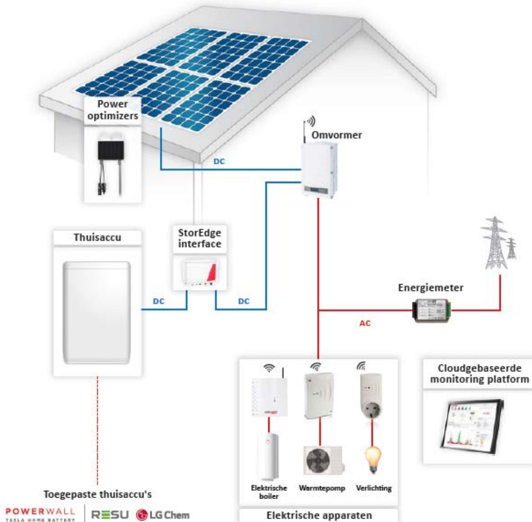
Afbeelding 1: Device Control systeemoverzicht
