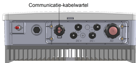
Afbeelding 12: Communicatie-kabelwartel
