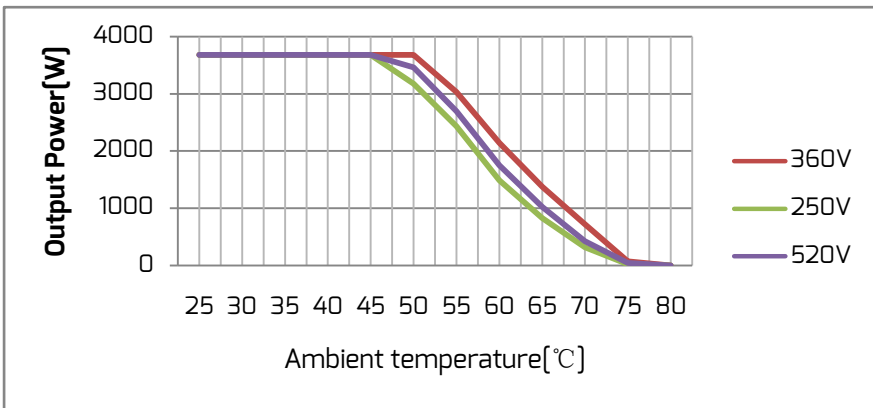
Vermogensreductie bij verhoogde omgevingstemperatuur (TL3680)
