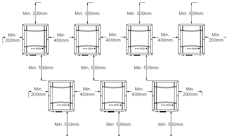
Afstanden bij meerdere omvormers
