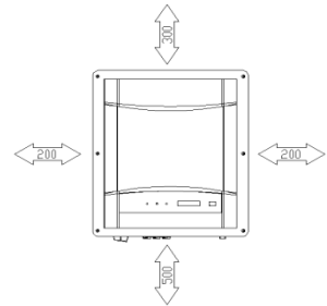
Afstanden bij 1 omvormer
