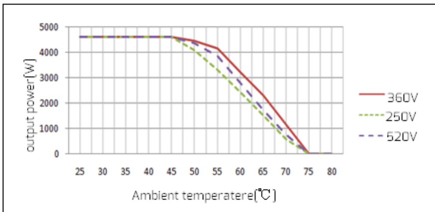
Vermogensreductie bij verhoogde omgevingstemperatuur(TL5000-10)
