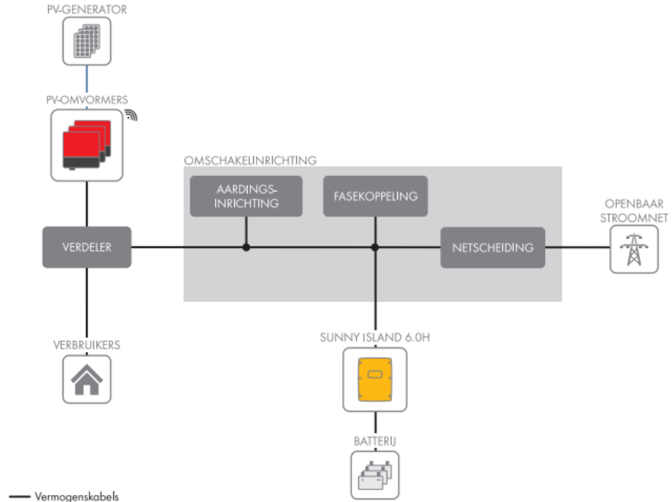
Afbeelding 1: Blokdiagram van een eenfasig noodstroomstelsel
