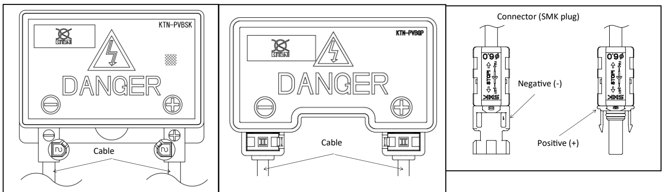
Figuur 2. Configuratie van aansluitdoos
