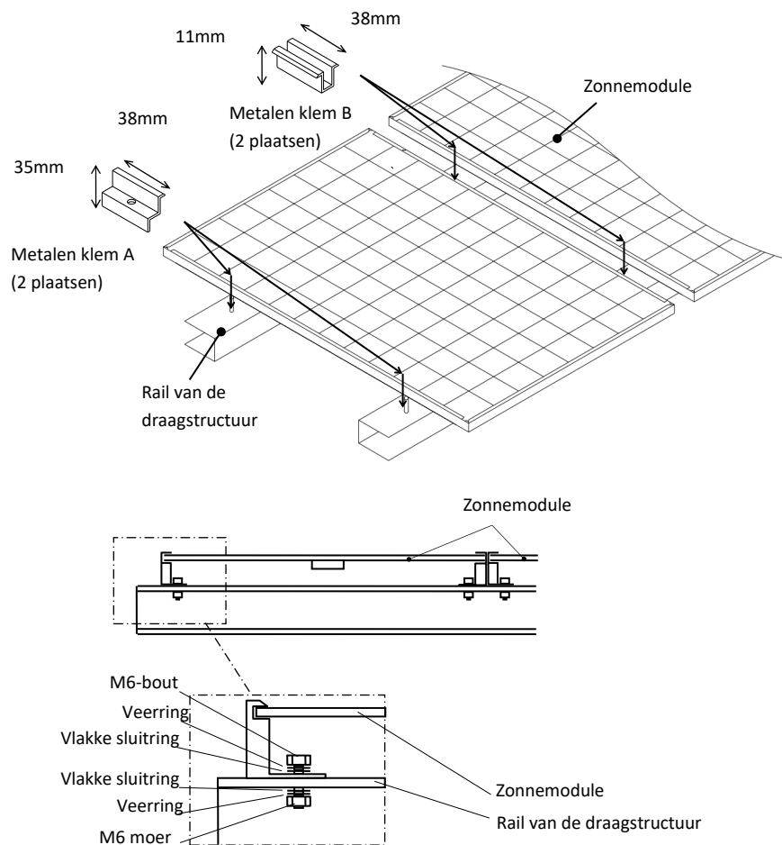
Figuur 5-1. Installatie van modules (VBHNxxxSJ25)
