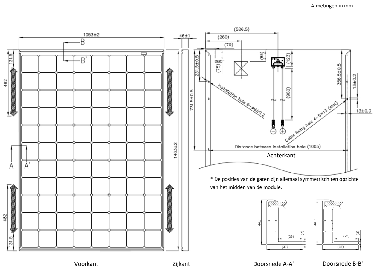
Figuur 1-2. Afmetingen van module (VBHNxxxSJ40)
