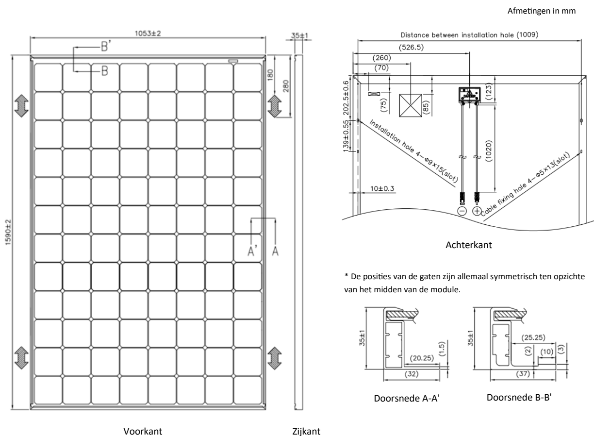
Figuur 1-4. Afmetingen van module (VBHNxxxSJ47)
