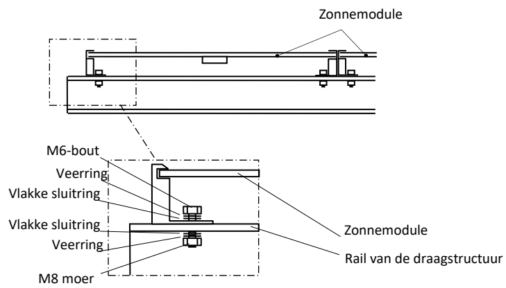
Figuur 5-2. Installatie van modules (VBHNxxxSJ40)
