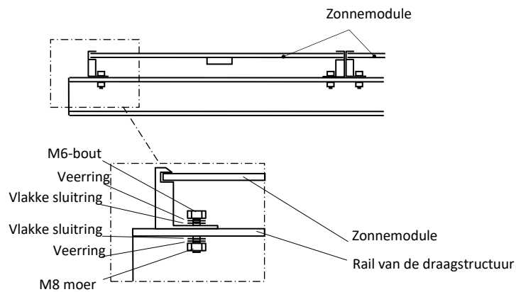
Figuur 5-3. Installatie van modules (VBHNxxxSJ46, VBHNxxxSJ47)
