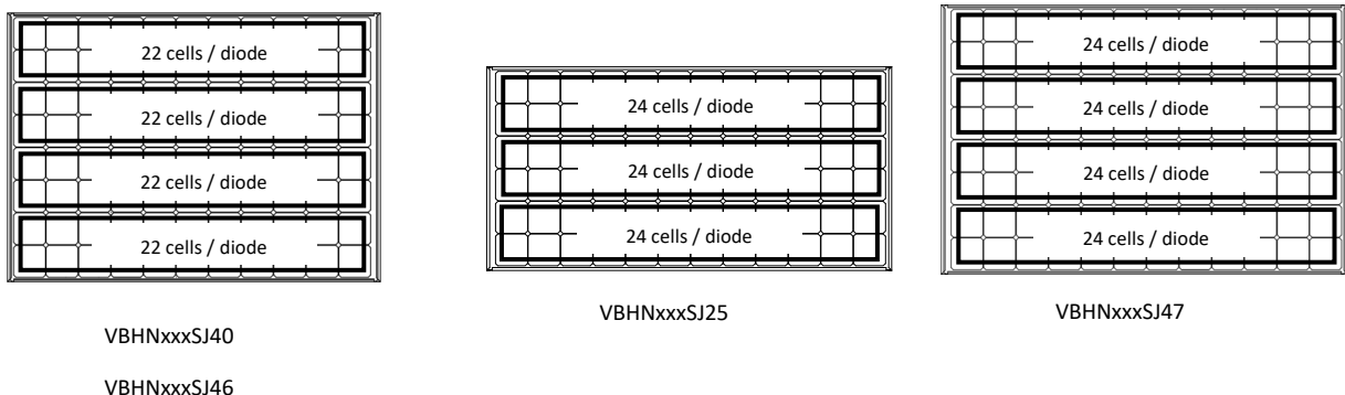
Figuur 3. Aantal cellen in serie per omloopdiode
