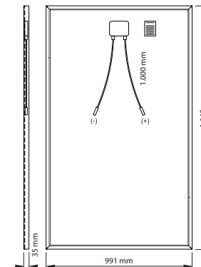
BISOL Spectrum paneel met standaard kader
