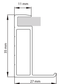
Doorsnede standaard kader
