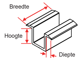
<Middelste klem>
