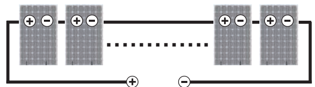
Raccordement en série pour obtenir davantage de tension
