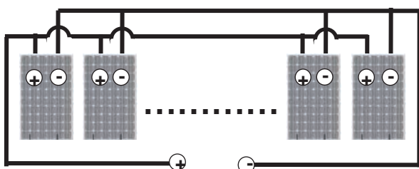
Raccordement en parallèle pour obtenir davantage de courant
