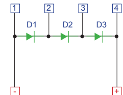
Spécification des diodes et configuration
