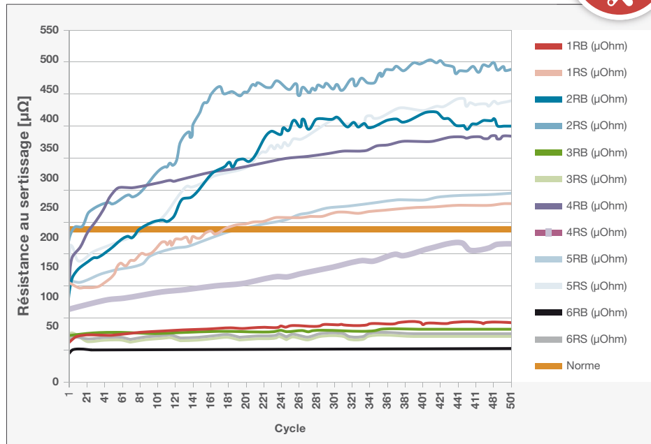
Illustration 8: Diagramme des forces de résistance du sertissage.
