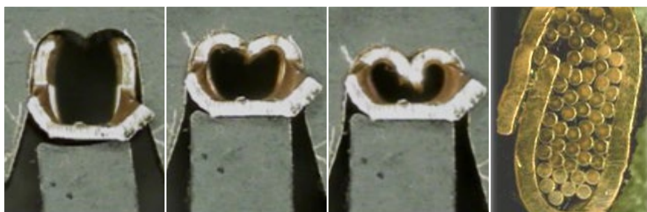
Le cylindrage de la zone de sertissage n'est pas uniforme
