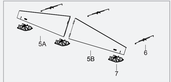
5. FlatFix Wave Déflecteur de vent A et B (= kit de déflecteur de vent) 1009103
