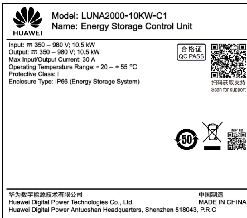
Afbeelding2-11 Typeplaatje van een besturingseenheid voor energieopslag
