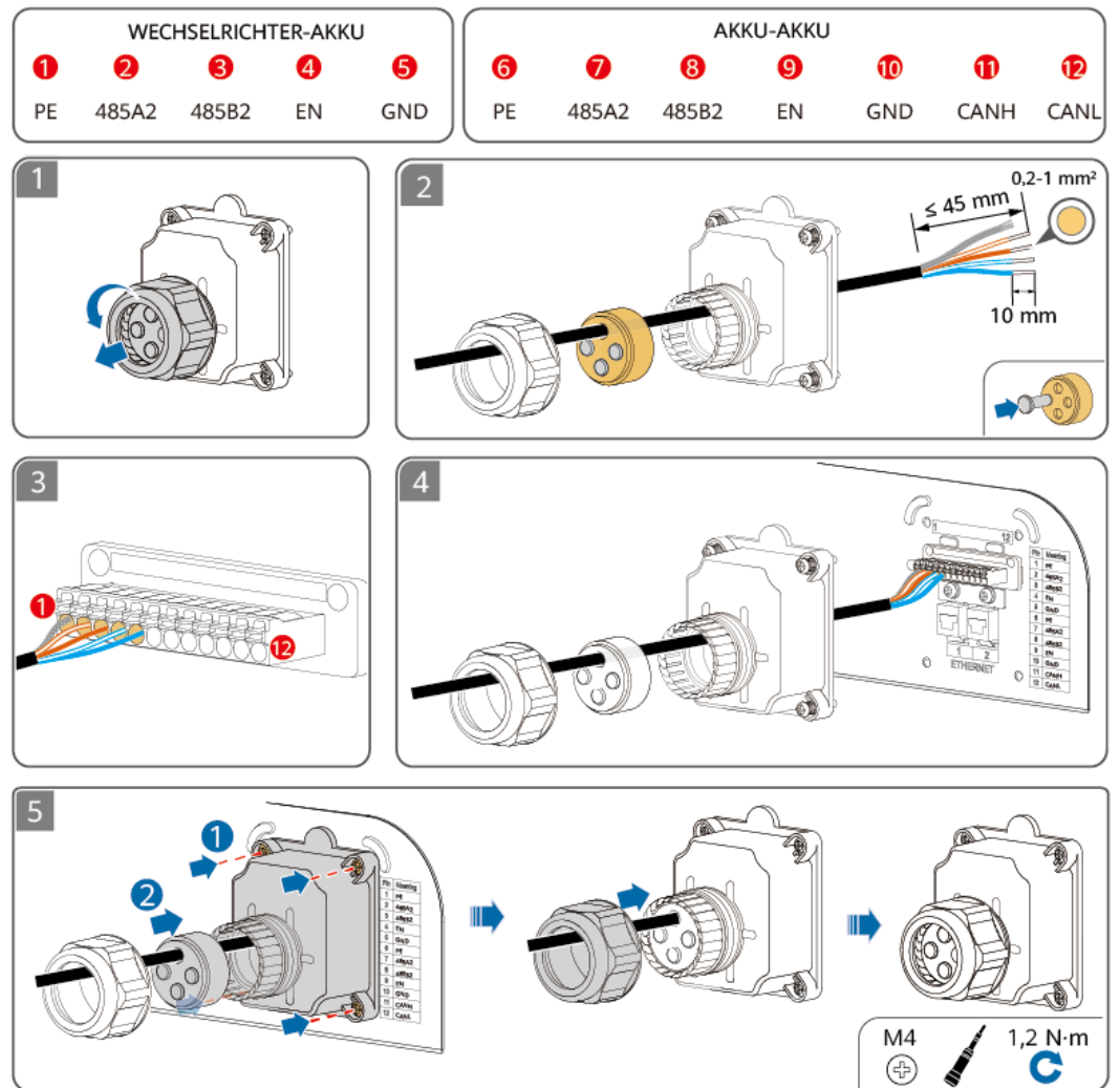
Afbeelding5-6 Signaalpoortaansluitingen
