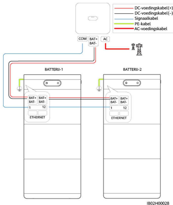
Afbeelding3-1 Kabelaansluitschema
