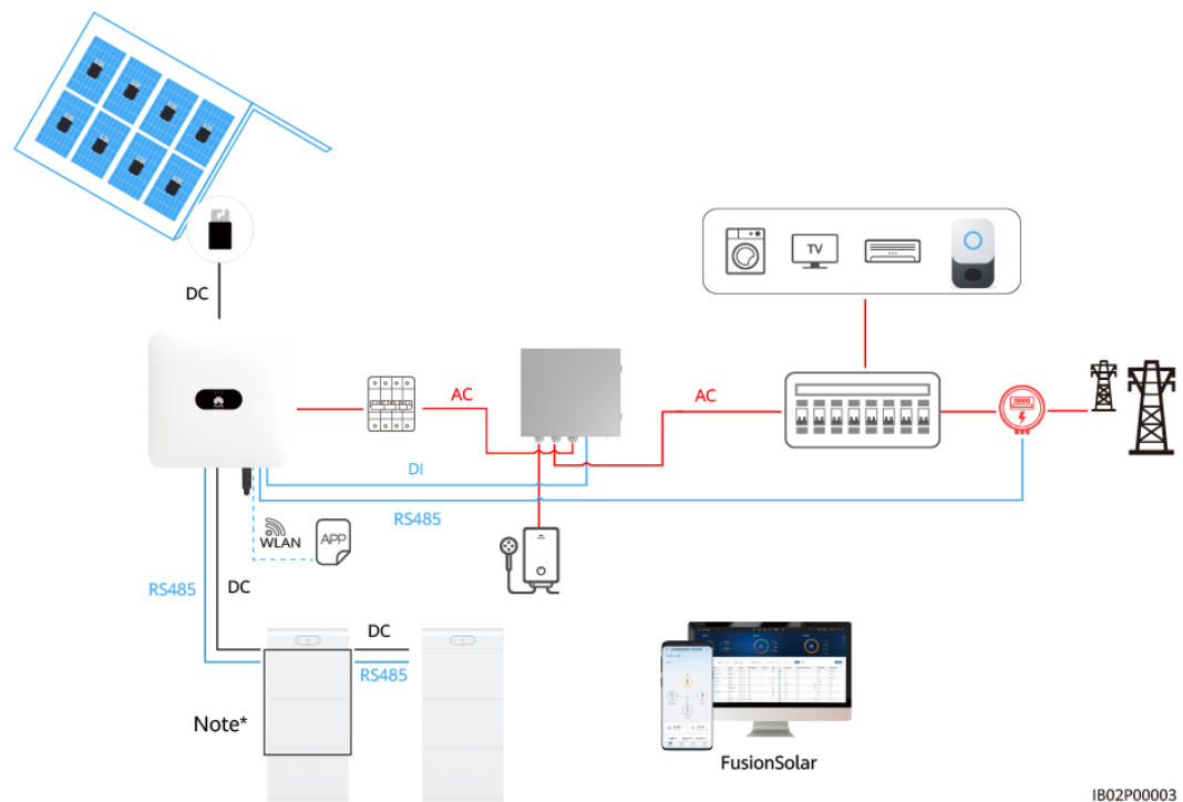
Afbeelding2-8 Via/niet via het net-scenario
