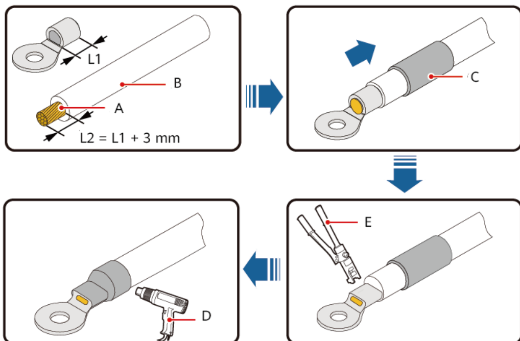
Afbeelding5-2 Een OT-aansluiting krimpen
