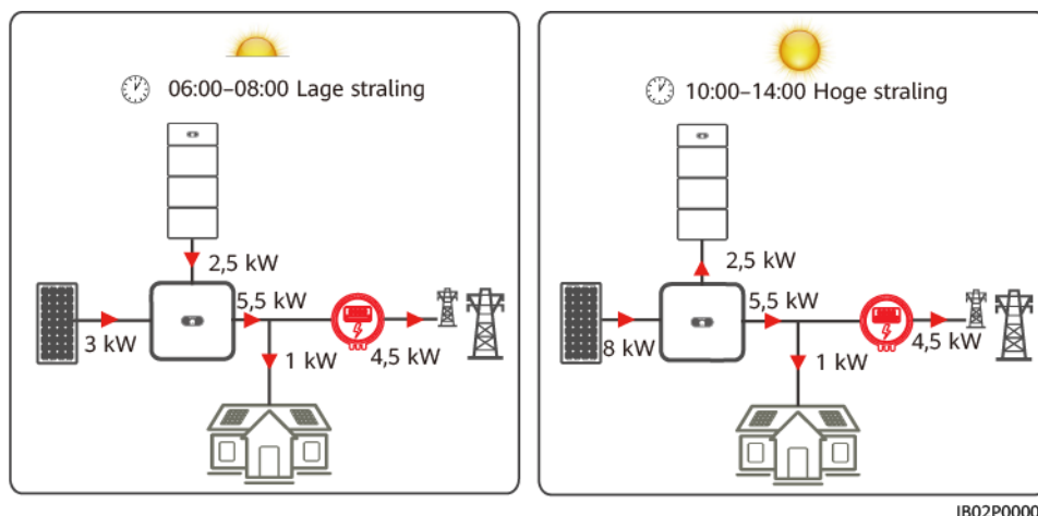
Afbeelding2-10 Volledig geleverd aan net
