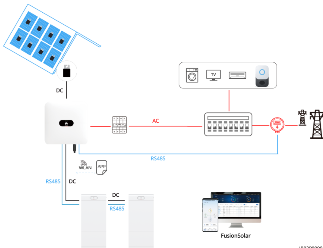
Afbeelding2-7 Via het net-scenario
