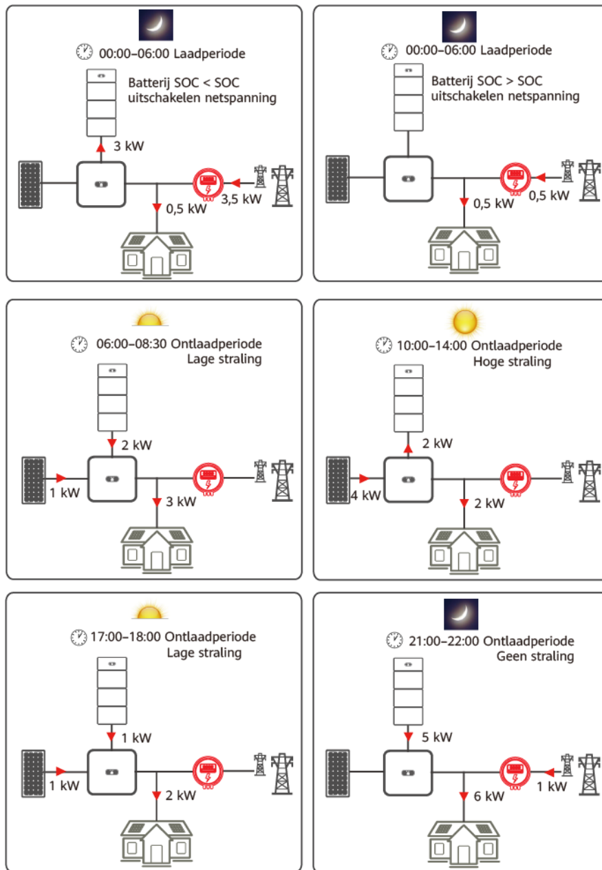
Afbeelding2-9 Voorbeeld van TOU (00:00–06:00 opladen en 6:00–24:00 ontladen)
