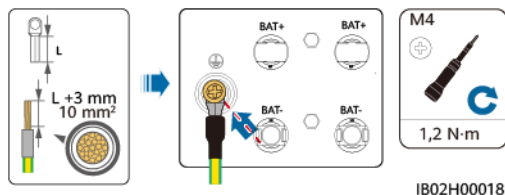
Afbeelding5-3 De PE-kabel aansluiten
