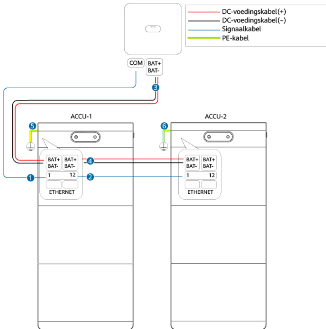
Afbeelding5-1 ESS-kabelaansluitingen
