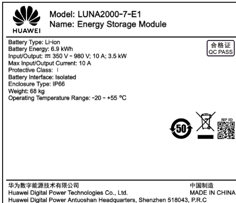
Afbeelding2-12 Typeplaatje van een energieopslagmodule
