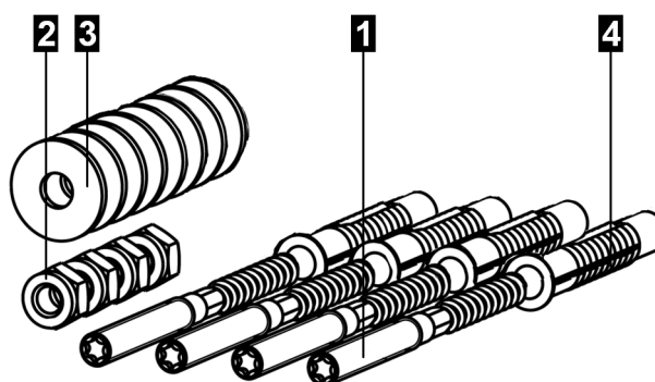
Afb. 3-3: Bevestigingsset voor muurmontage
