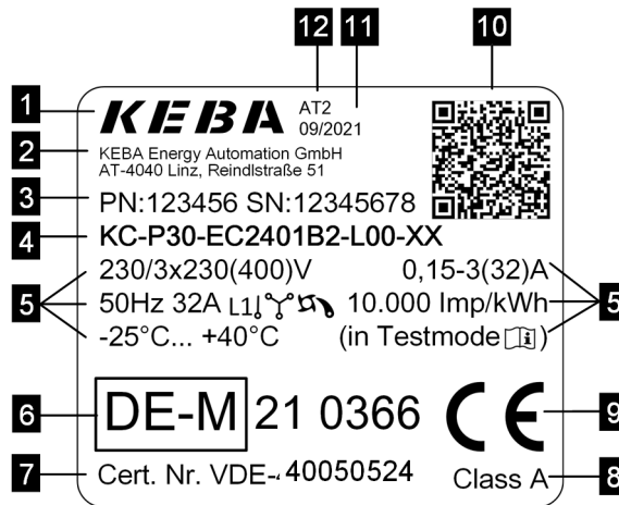
Afb. 4-7: Typeplaatje (voorbeeld)
