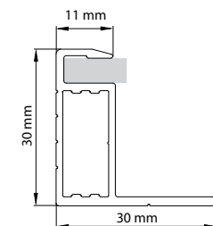
Doorsnede standaard kader
