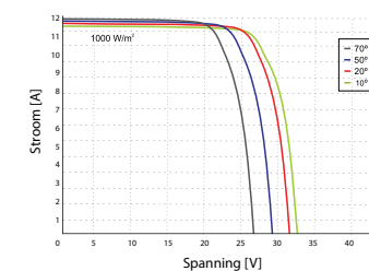
I-V Curve bij verschillende celtemperaturen
