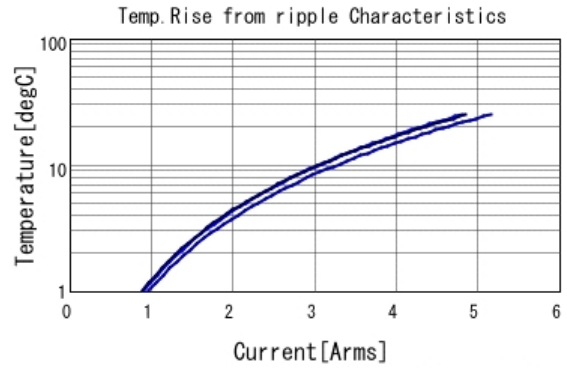
KRM55WR71E476MH01 Temp. rise ■ 50kHz ■ 100kHz ■ 300kHz
