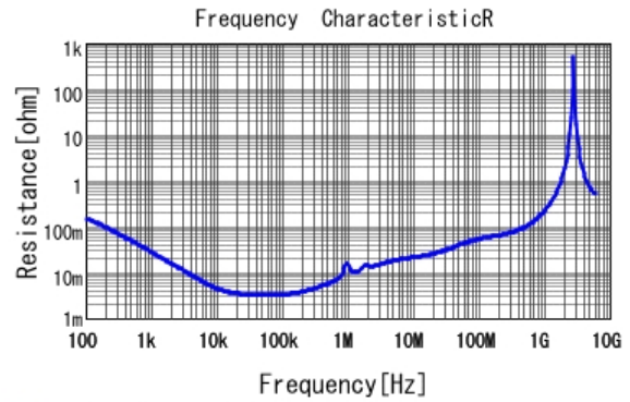
■ KRM55WR71E476MH01 R DCOV, 25degC
