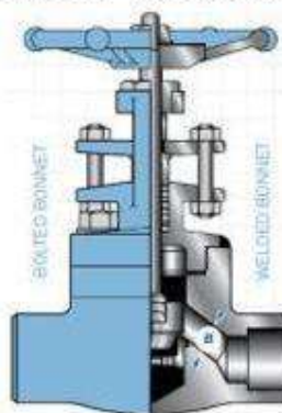
B) GLOBO FORJADA
