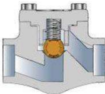
D) RETENCION BOLA FORJADA
