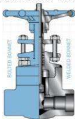
A) COMPUERTA FORJADA
