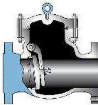
J) RETENCION COLUMPIO FUNDIDA
