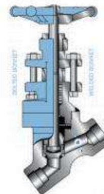
C) GLOBO "Y" FORJADA
