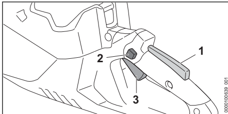
Palanca Ergo (1), bloqueo del gatillo (2) y gatillo (3)
