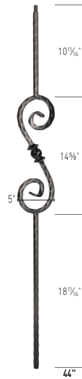
310 44 1/2" Hammered Edge
