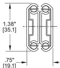
301 175 lbs./pr. [80 kg]
