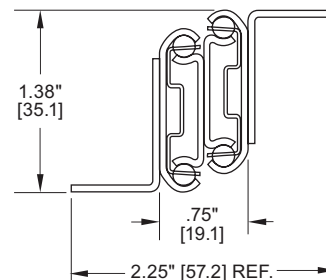
301-2590 155 lbs./pr. [70 kg]
