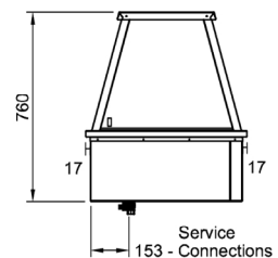
End Elevation
