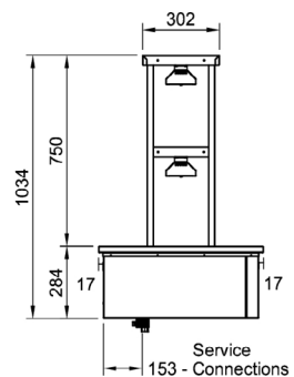
End Elevation
