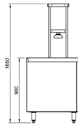
End Elevation
