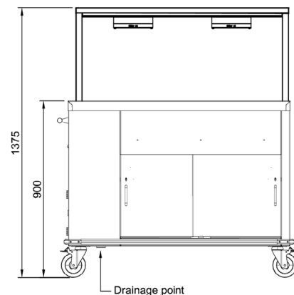
End Elevation
