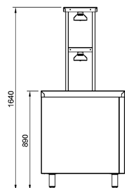
End Elevation
